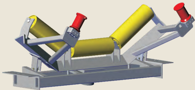
升程式调心托辊组 Riser aligning idler set
