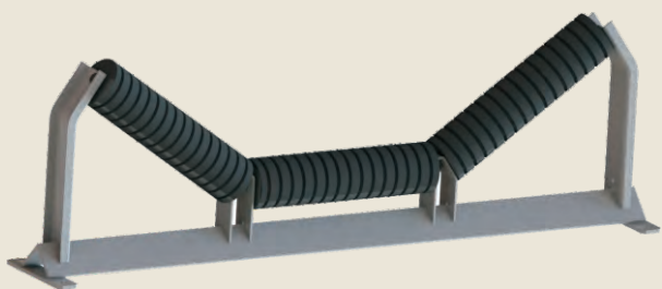
普通缓冲托辊组 Normal impact idler
